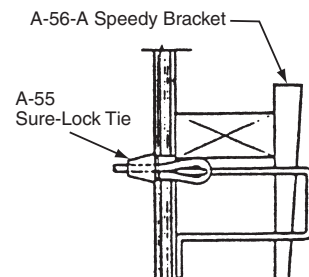
A-56-A Speedy Bracket
